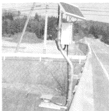
鳥谷川の危機管理型水位計
