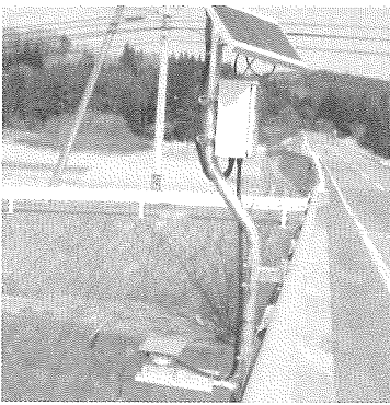
鳥谷川の危機管理型水位計
